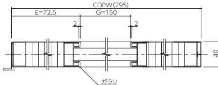
F-F'
