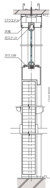
D-D'
