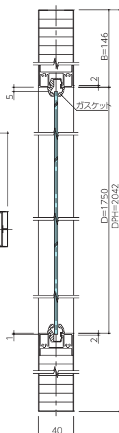
B-B'
