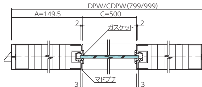
D-D'
