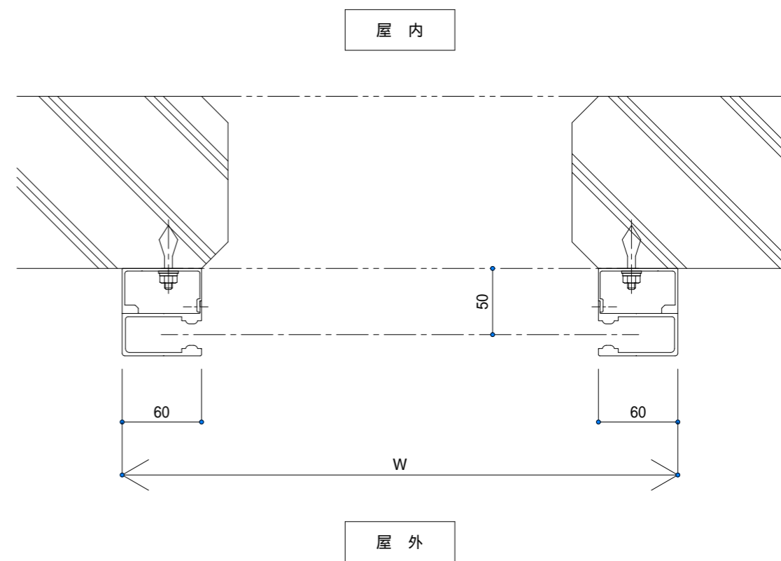
本図はP型ケース（手動式）外巻き：納まり詳細図
