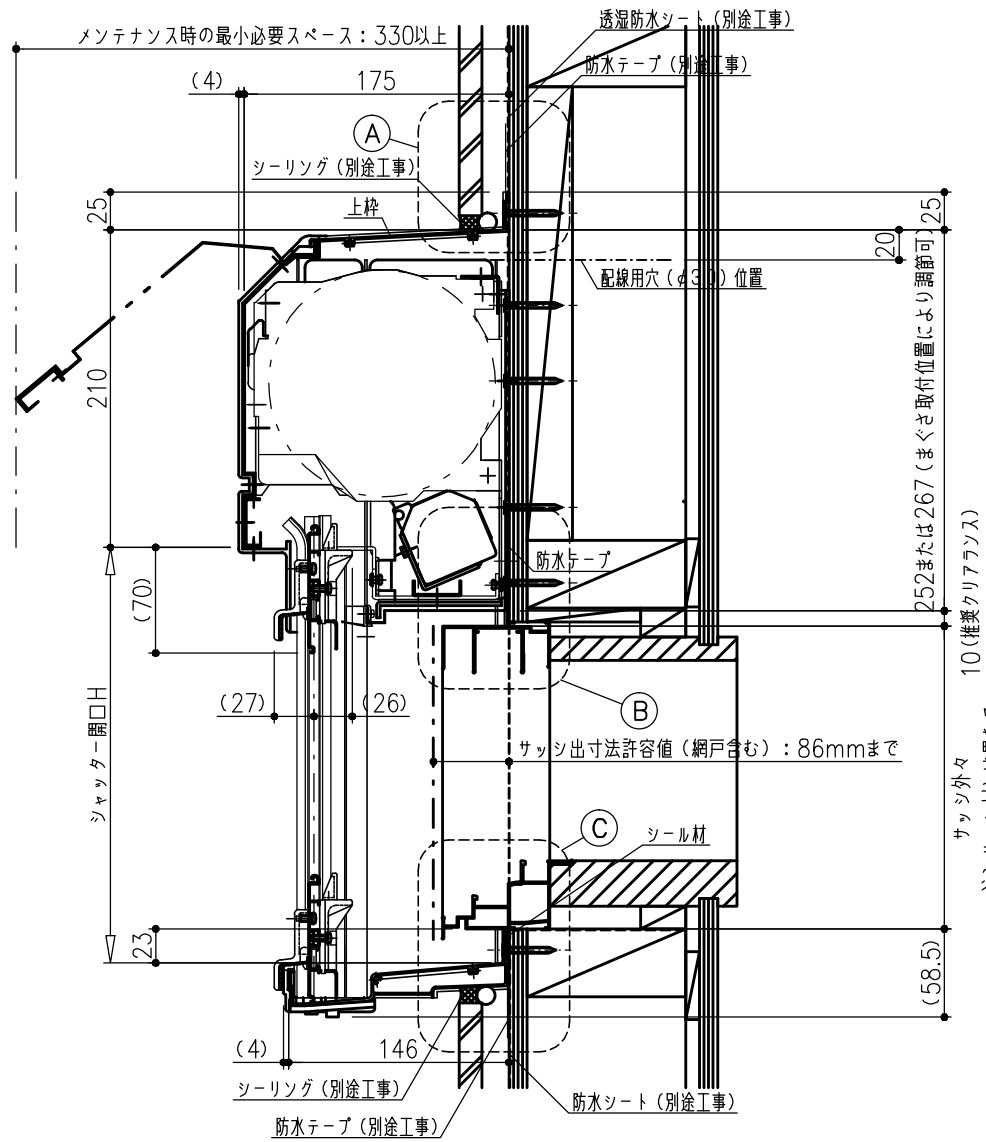
縦断面図
