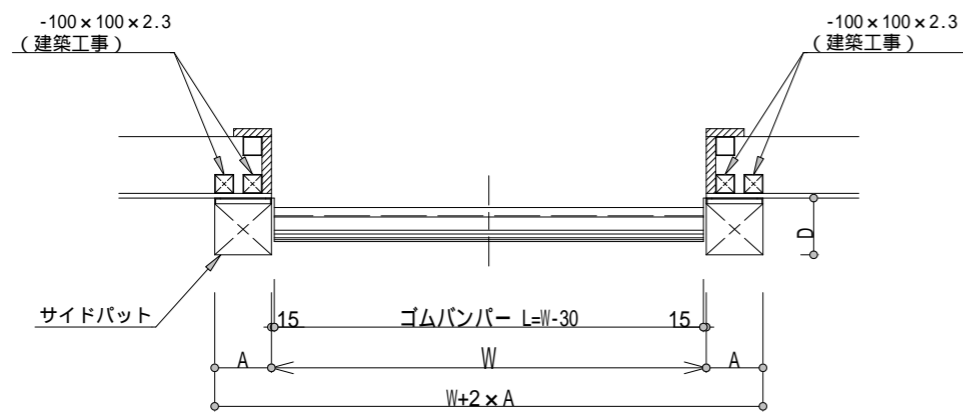
平面図
