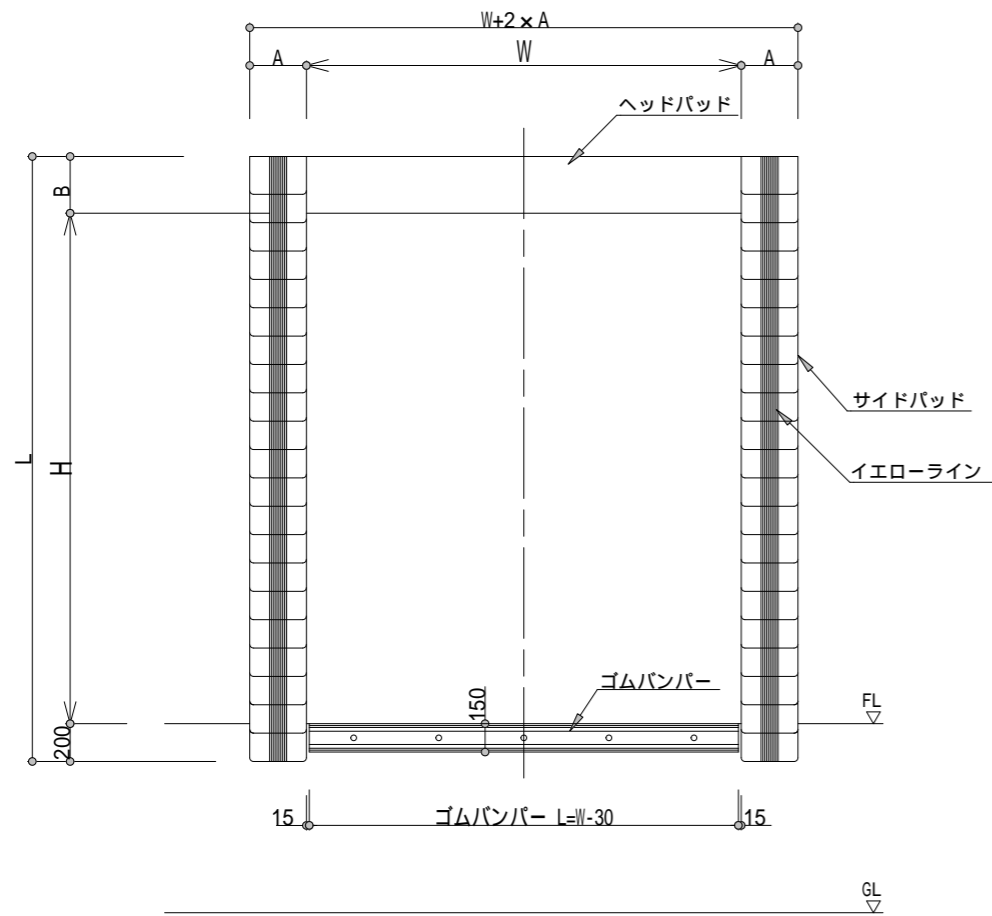
正面図
