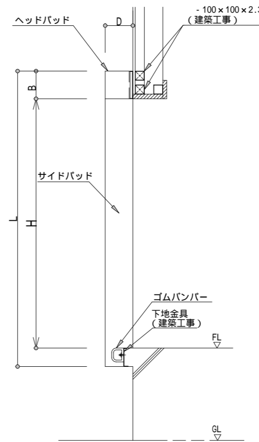
断面図
