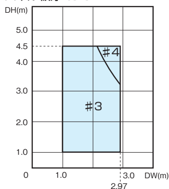
パネル板厚 t0.8
