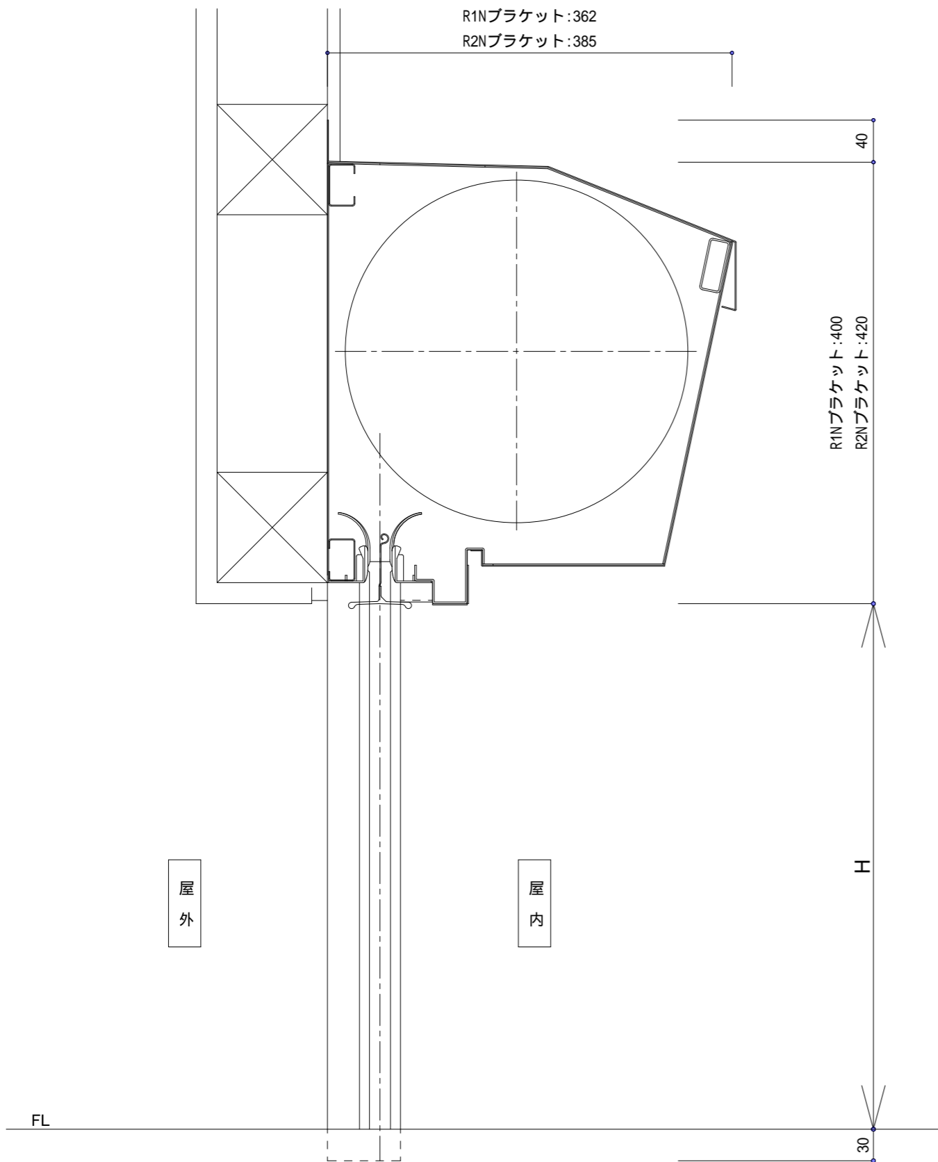
縦断面納まり図（内巻き）
