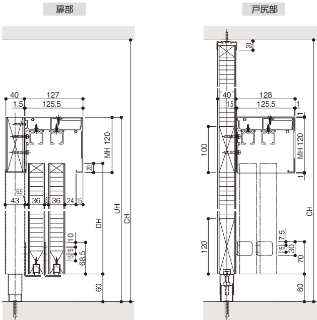
縦断面図
