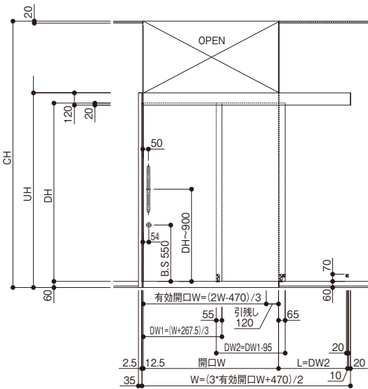
内観図
