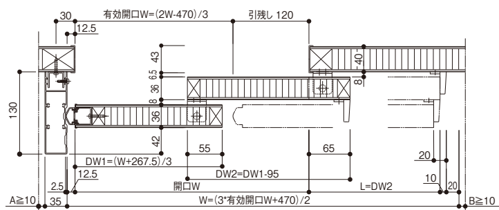
■横断面図
