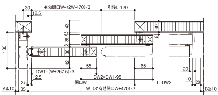
横断面図
