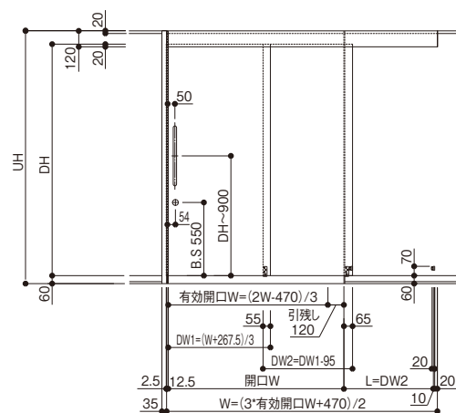
■内観図
